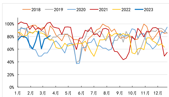
图 48: TDI 周度开工负荷
