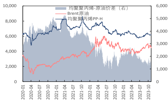
图 33: 原油、均聚聚丙烯价格及价差 (元/吨, 元/吨)
