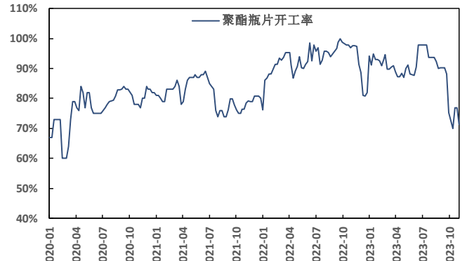
图 60: 2020-2023 年聚酯瓶片开工率 (%)
