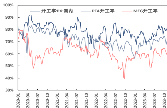
图 41: PX、PTA 和 MEG 开工率 (%)
