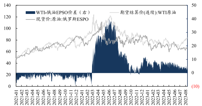
图10: WTI、ESPO 原油价格及价差 (美元/桶, 美元/桶)
